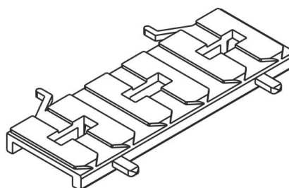
Cam Takoza Glass Wedge (Thick) Подкладка стеклопакета تسميكة الزجاج
