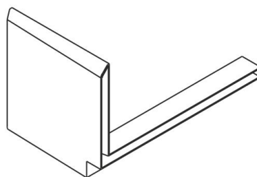
80x150 Pervaz Rozeti 80x150 Cornice badge 80x150 Соединитель профиля откоса وصلة تشبيك الكشف ٨٠x١٥٠
