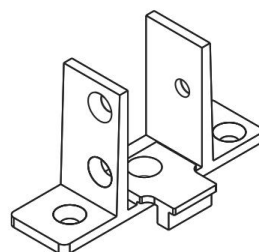
KOM 500 Ortakayıt Bağlantı Takoza KOM 500 Mullion fitting wedge Kom 500 Держатель импоста لقمة تي كوم ٥٠٠
