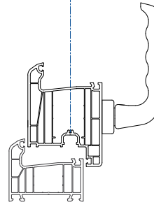
M5 tipinde tek taraflı kol ve rozet kullanılmaktadır
