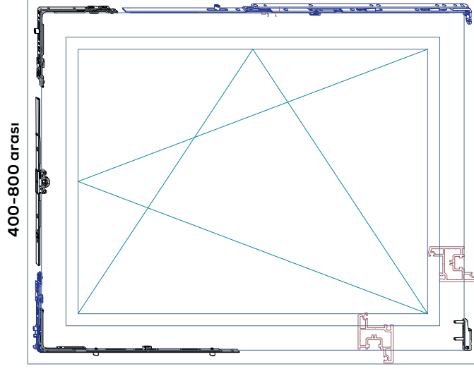
Geniş Kısa Pencere 800-1600 arası
