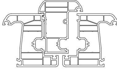
Profil Tip 3
