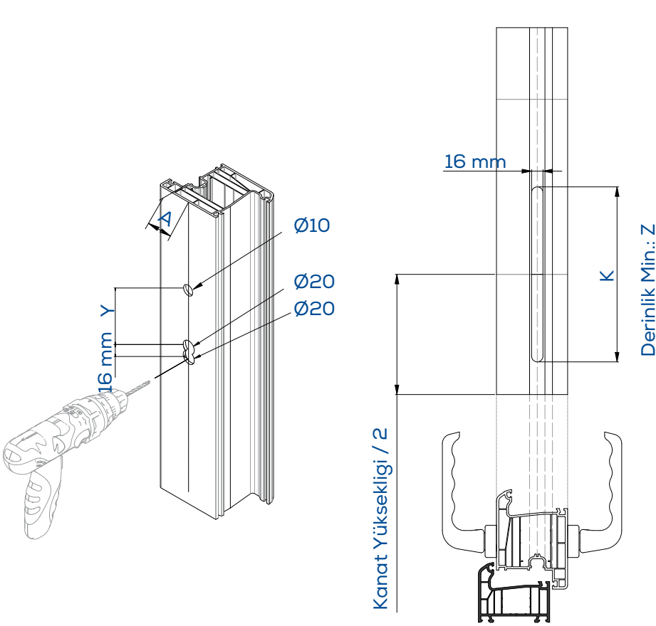
Aral Kesilebilir Sürgülü Kol Yeri Hazırlama WK
