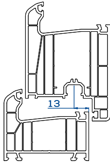
Profil Tip 3
