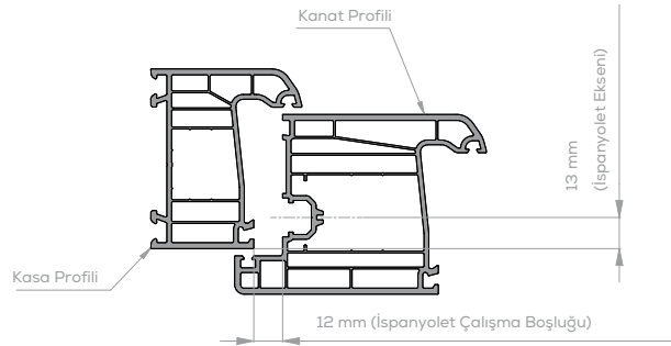
Kapı Kanat Kasa Uygulaması
