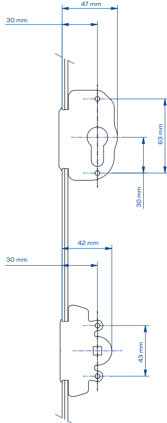
M5 tipinde tek taraflı kol ve rozet kullanılmaktadır
