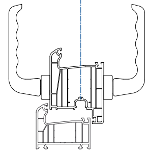
Ø5 tipinde tek taraflı kol ve rozet kullanılmaktadır
