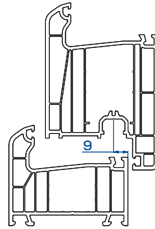
Profil Tip 4
