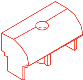
Kanat Kaldırma Takoza (Kanada Montaj) Lifting Wedge for Sash (Mounting to Sash) Фиксатор-балансир створки ترفيعة الضلفة (يركب على الضلفة)
