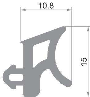
17mm cam contaı Glass joint for 17 mm 17 мм уплотнитель стекла جوان للزجاج ١٧مم
