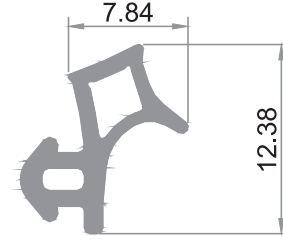
Kasa-kanat contaı Frame-Sash Joint уплотнитель рама-створка جوان للإطار والصففة
