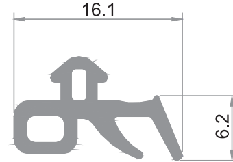
18mm Universal conta Universal Joint for 18 mm 18 мм Универсалный уплотнитель جوان أونى وارسلال ١٨مم
