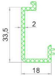
Eşik Kapama Profili Threshold Cover Profile Профиль порога بروفيل غطاء الكادر
