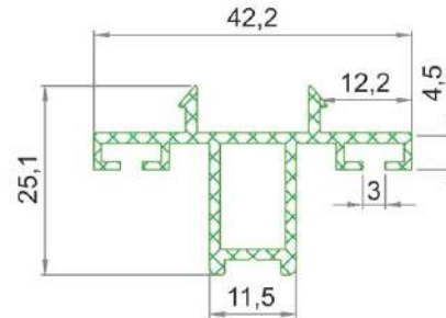
Ara Kilitleme Profili Sliding Locking Profile Профиль среднего запираания بروفيل قفل داخلي
