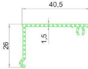
Geniş Kanal Kapama Profili Large Slot Cover Profile Широкий облицовочный профиль канала بروفيل غطاء القناة العريضة
