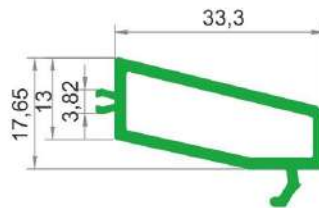
Kom 819 / ٨١٩ Eşik Kapama Profili Threshold Cover Profile Профиль порога بروفيل غطاء الكادر
