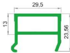
Kom 818 / ٨١٨ Geniş Kanal Kapama Profili Large Slot Cover Profile Широкий облицовочный профиль канала بروفيل غطاء القناة العريضة
